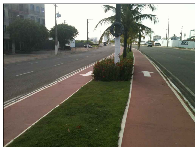
DETALHE IMPLANTAÇÃO DE CICLOFAIXA EM CANTEIRO CENTRAL
